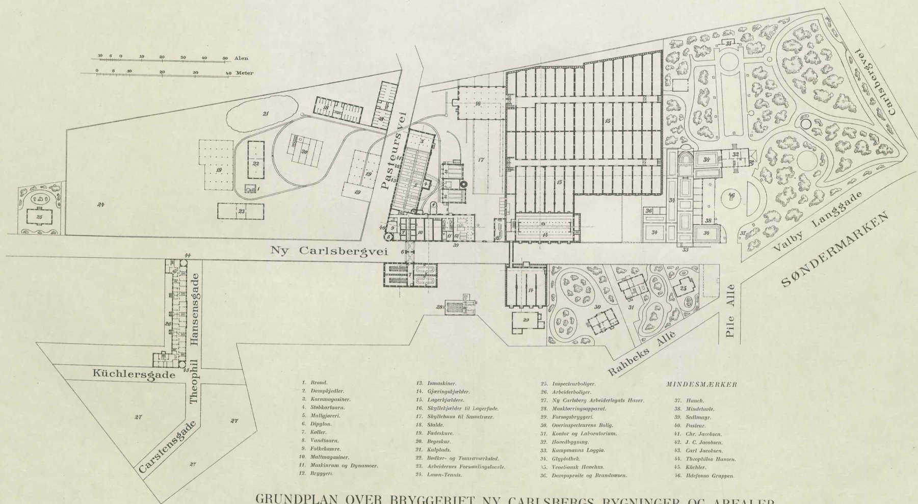
GRUNDPLAN OVER BRYGGERIET NY CARLSBERGS BYGNINGER OG AREALER.
