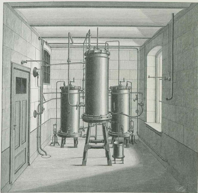
Dr. E. Hansens Reengjersapparat.
