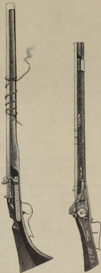
Fig. 9. Luntebøssen. Fig. 10. Karabinen.
