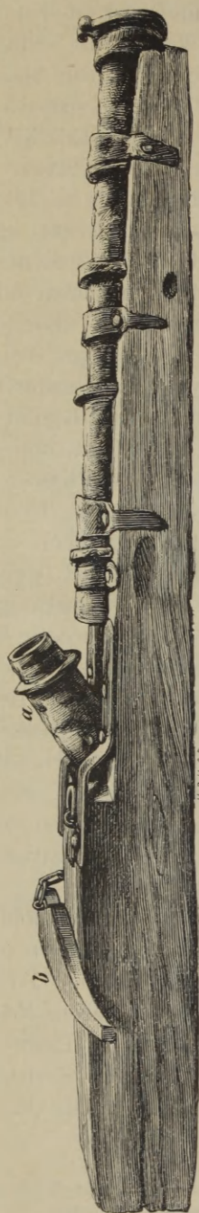
Fig. 3 a. Bagladekanon 1. Aar 1400. a løst Kammerstykke med Krave til Krudtladning. b Kile, der fastholder Kammerstykket. Kanonens Underlag er en udhulet Træstamme.
