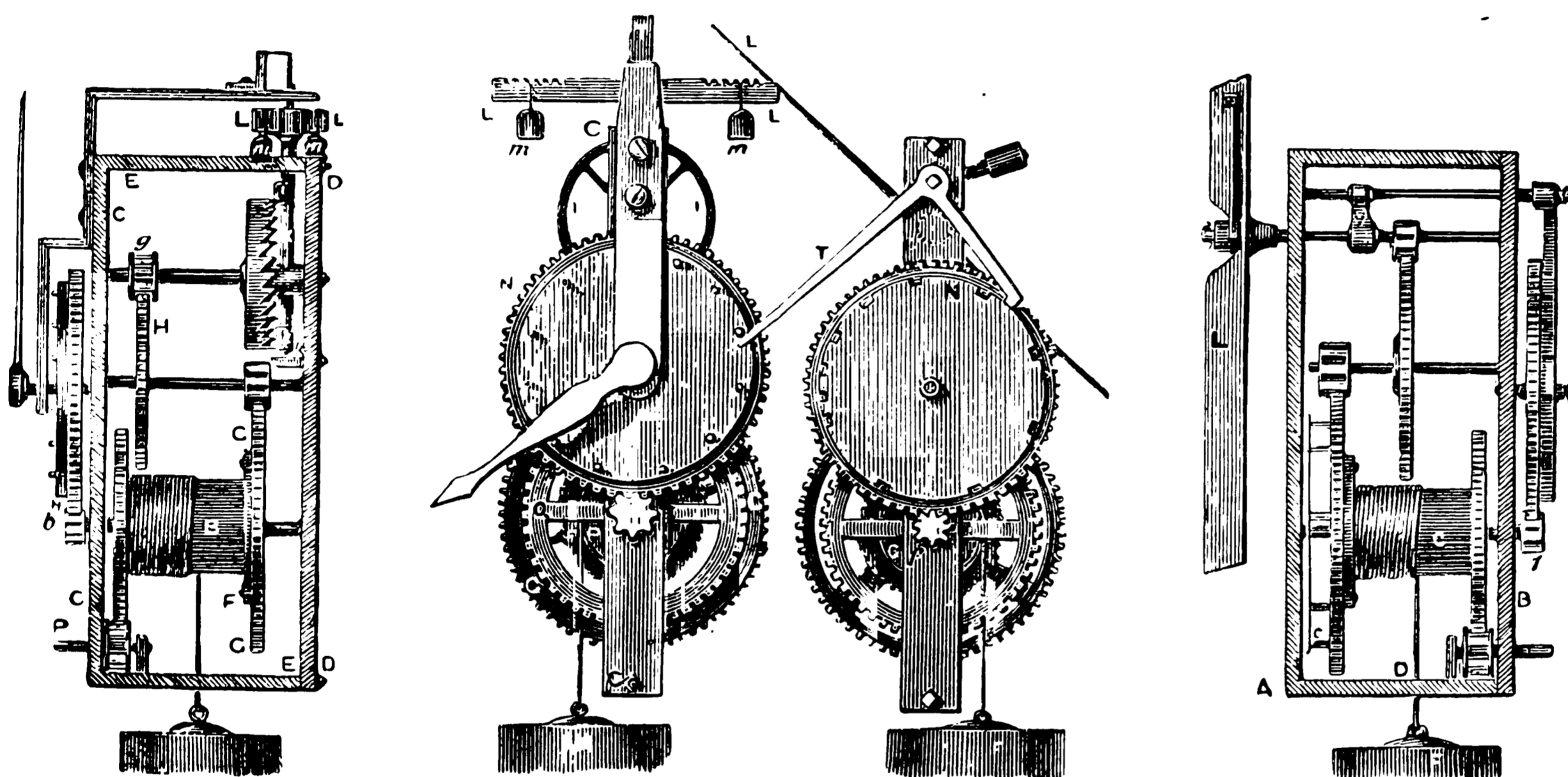
Slagur fra Palais-de-Justice i Paris, forfærdiget 1370 af Henri de Vick.
