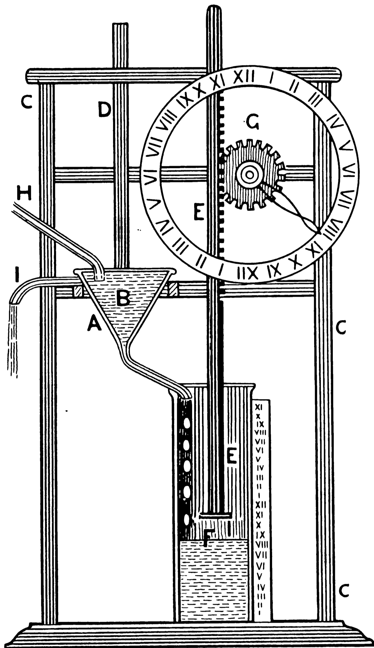
Rekonstruktion af et ægyptisk (?) Vandur fra Oldtiden. Talring og Skala er en senere Tilføjelse.
