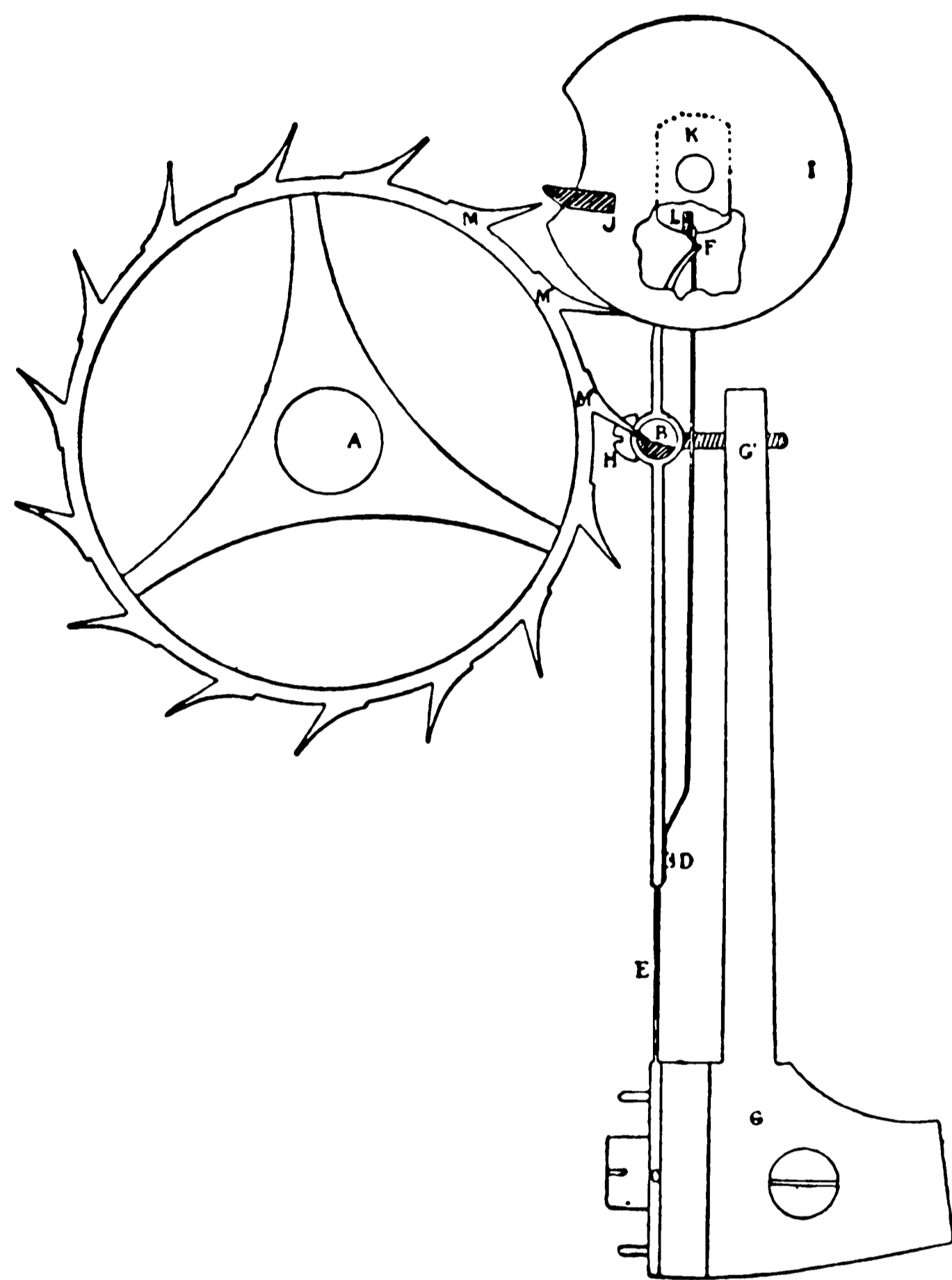
Kronometer- eller Fjedergang.
