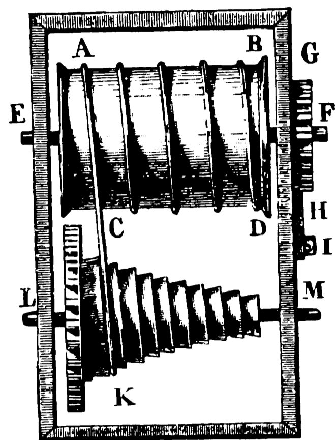
Snekke og Fjederhus.
