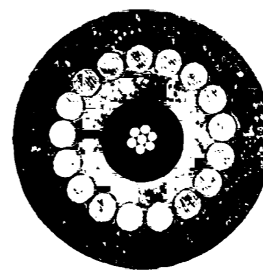
Almindeligt Hovedkabel i Øst-asien (2 Tons).
