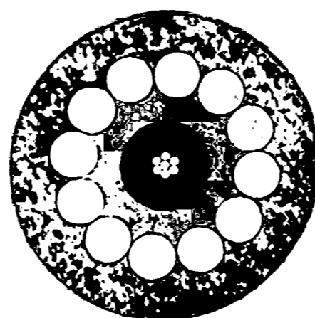
Almindeligt Hovedkabel i Europa ( 3\frac{1}{2} Tons).
