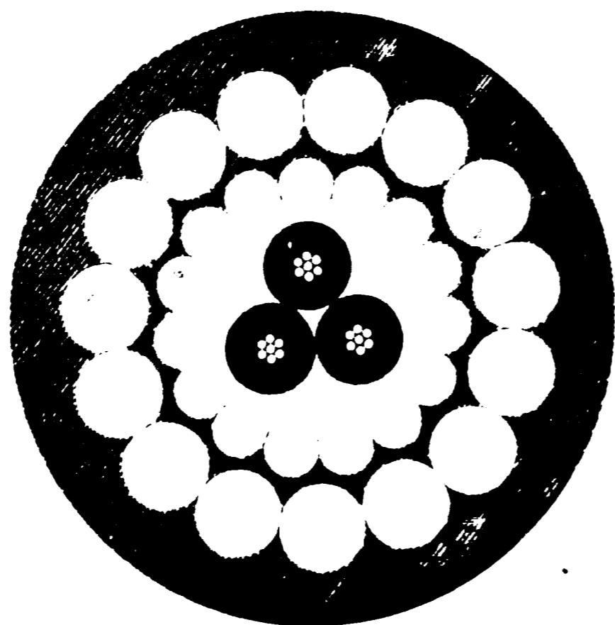
3-coret Woosung-Gutzlaff Flodkabel (17 Tons).
