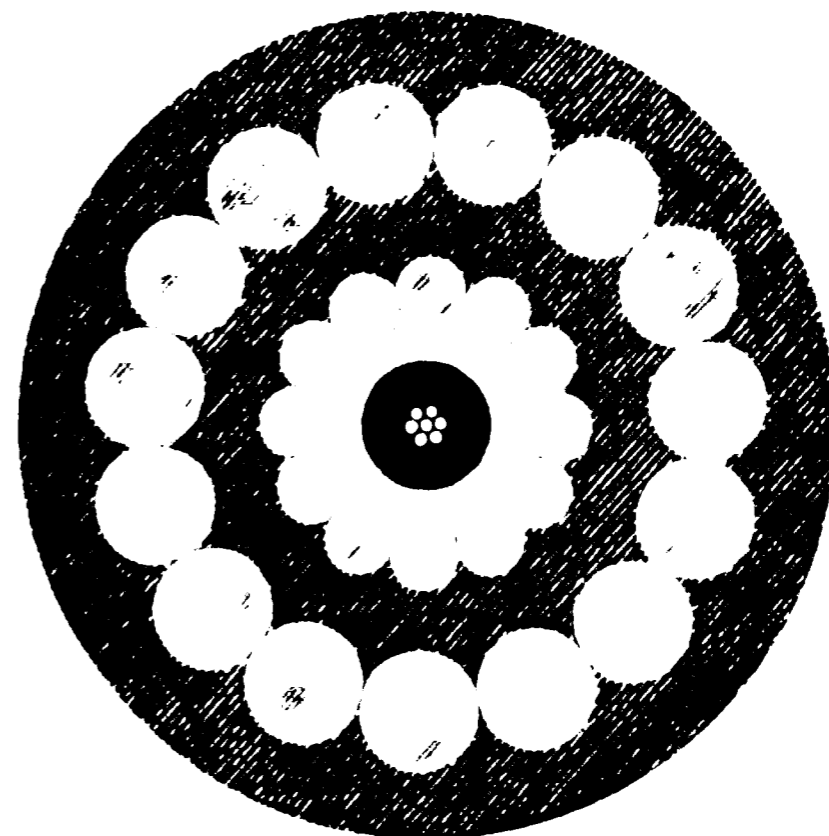
Svært Kystkabel (14 Tons).
